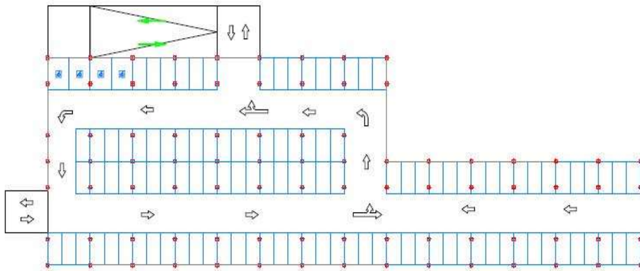
PLANTA BAJA 117 PLAZAS
