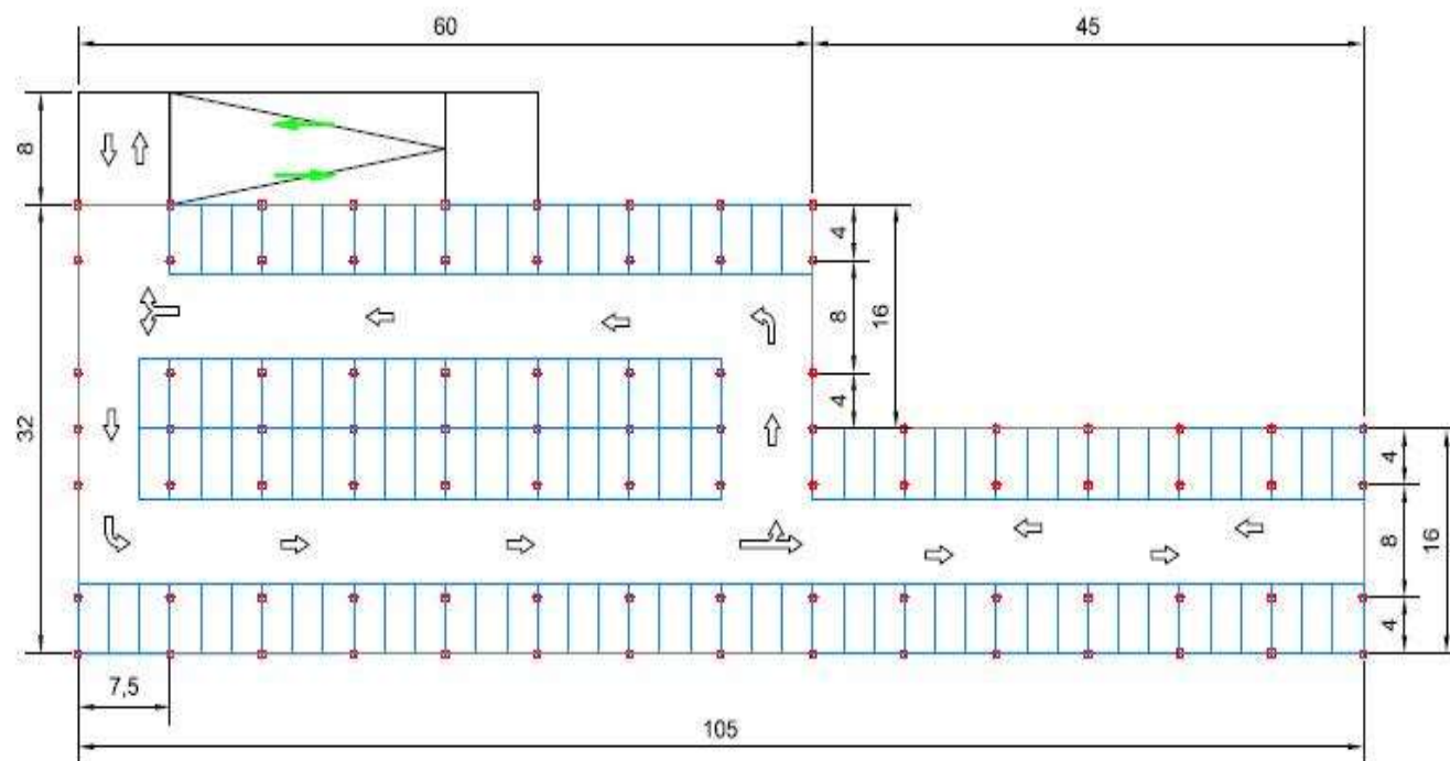
PLANTA PRIMERA 123 PLAZAS
